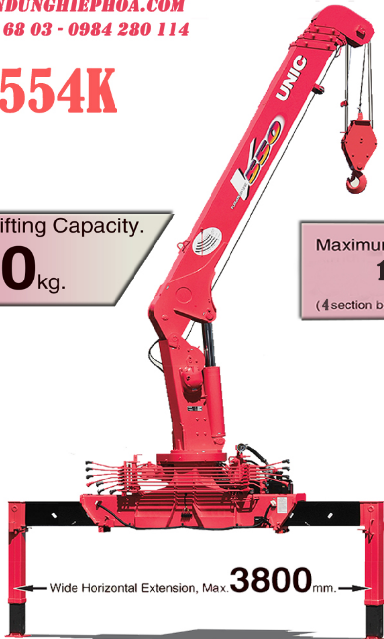
Model UR-V554K-TH với 4 đoạn cần
